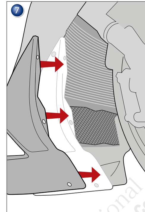
Protección del radiador del aceite Pieza 31961-002
