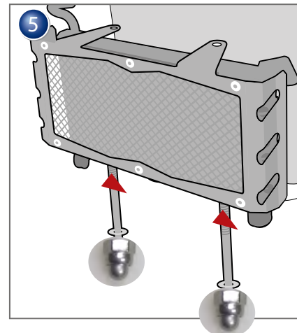
Protection de radiateur d'huile Pièce 31961-002
