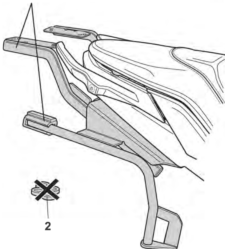
TOPCASETRÄGER X-RACK TOPCASE RACK X-RACK PORTE-BAGAGES SUPÉRIEUR X-RACK
