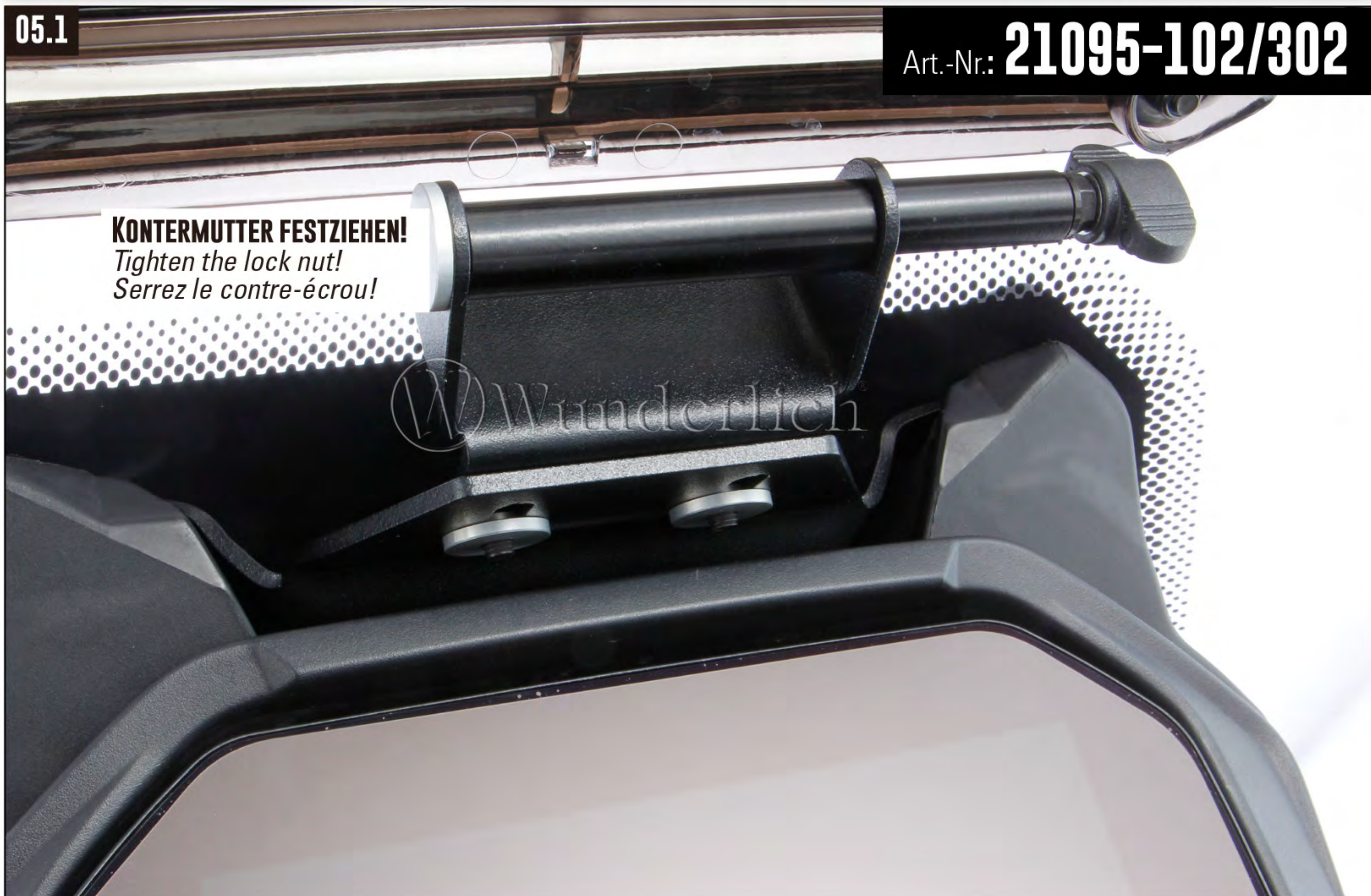
ANSCHLUß ORIGINAL NAVI. Connection of original navigation system. Connexion système de navigation d'origine.
